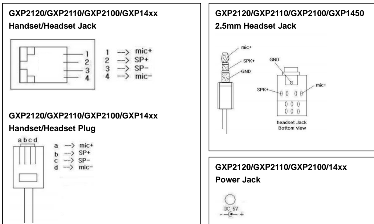
Figure 1: GXP2120/GXP2110/GXP2100/GXP14xx Pin-out
